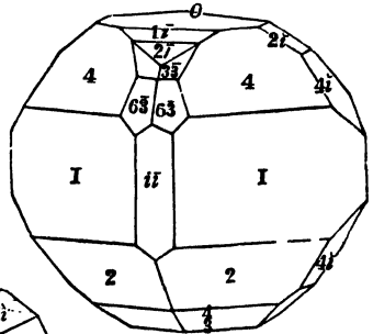
Isle Royale.
